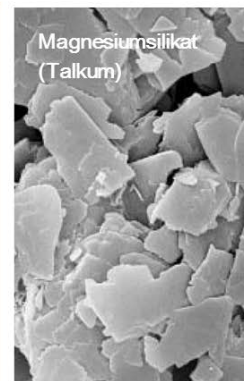
REM-Aufnahme von Talkum, 5000-fache Vergrößerung.
