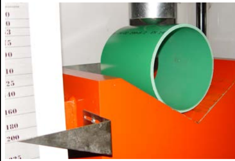
Bild: Kugelfalltest nach DIN EN 744
