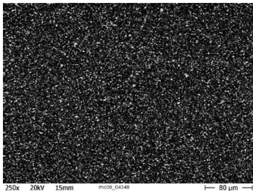
Bild 2: Homogene und feinste Verteilung des Verstärkungsmaterials Calciumcarbonat
