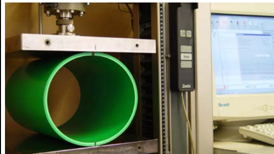
Bild: Prüfung der Ringsteifigkeit nach DIN EN ISO 9969
