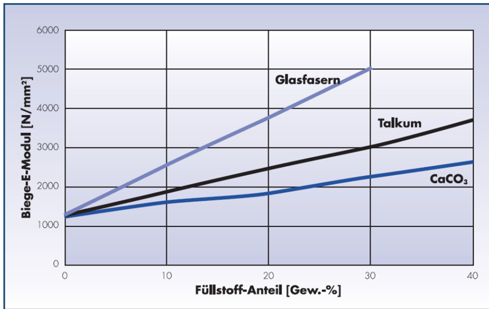
Bild: Biege-E-Modul von Polypropylen-Verbundwerkstoffe in Abhängigkeit von Gehalt und Formfaktor des Zusatzstoffes
