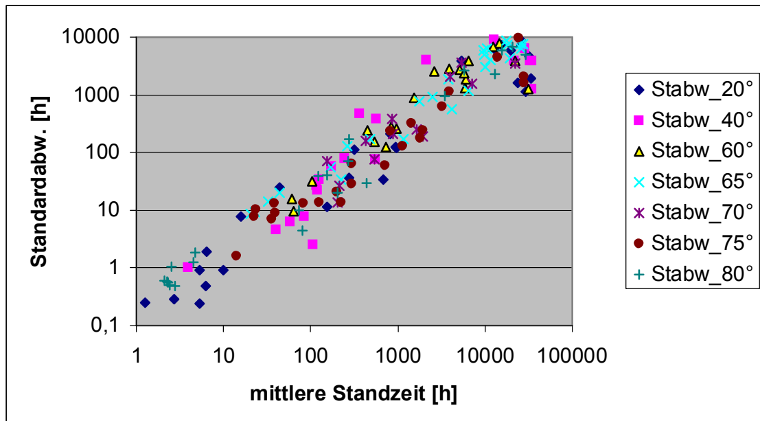
Bild 37: Streuung Zeitstand-Innendruckversuch
