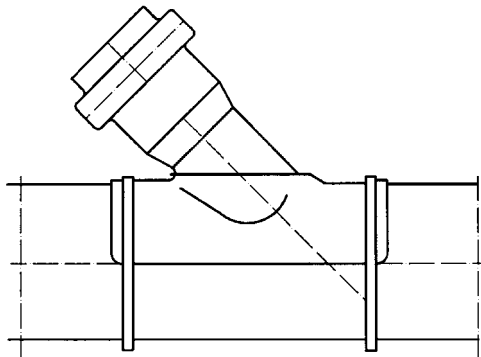
Bild 15: Klebschelle
