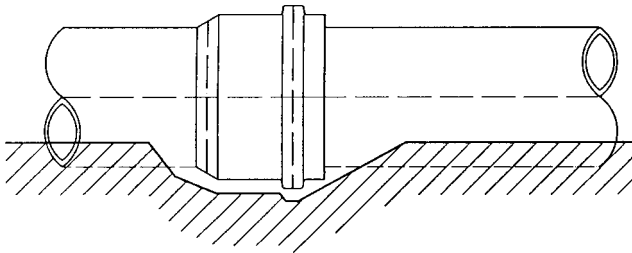
Bild 4: Muffenaussparung
