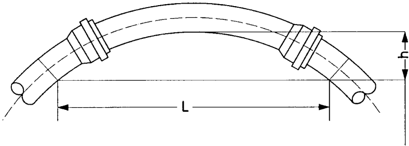
Bild 2: Gebogene Leitungsführung
