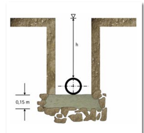
Bild 36: Herstellen der Grabensohle
