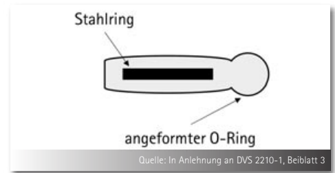
Bild 33: Querschnitt einer Profildichtung mit einvulkanisiertem Stahlring und angeformtem O-Ring
