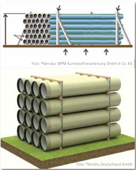
Bild 20: Lagerung nicht palettierter Rohre
