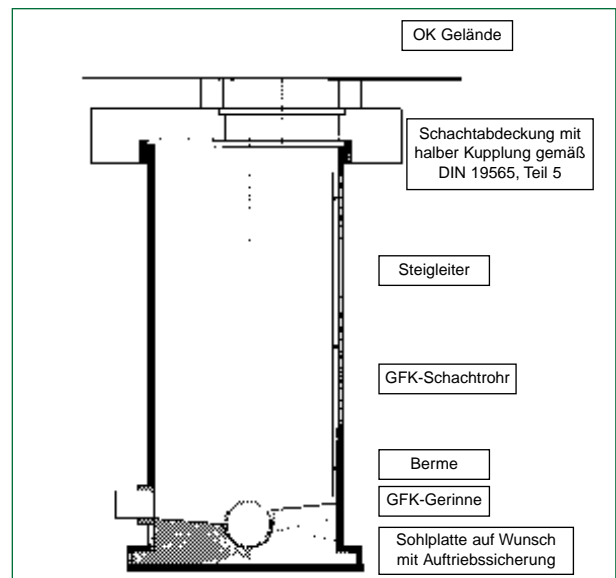
Bild 6: GFK-Schacht (Beispiel)
